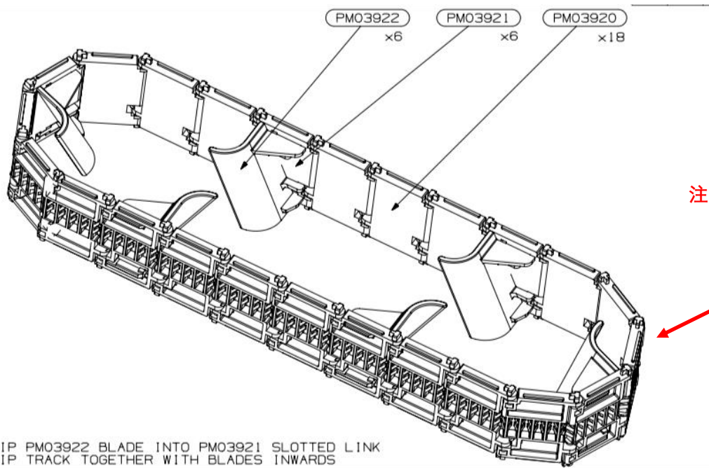
图一, 六个 PA04405-1 组件。
