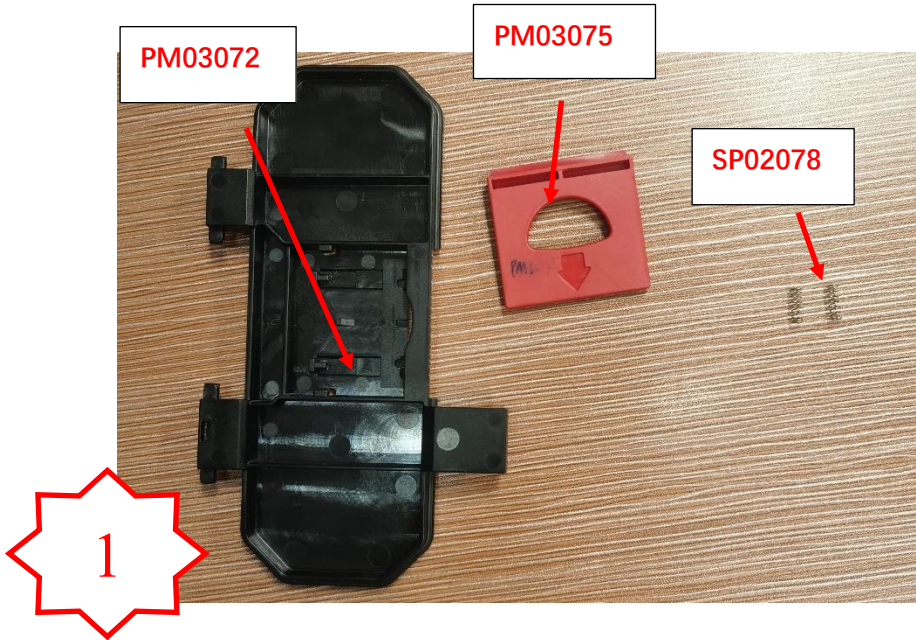
图一, 物料识别 PM03072, PM03075, SP02078。
