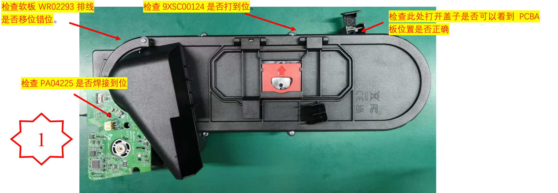
图一，目检 PA04401-3 组件。
