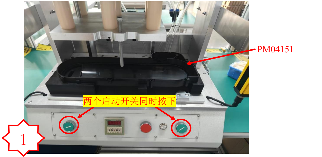
图一, 将 PM04151 放入自动点油机, 并同时按下两个启动开关。(PM04152 点油也按照此步骤进行)
