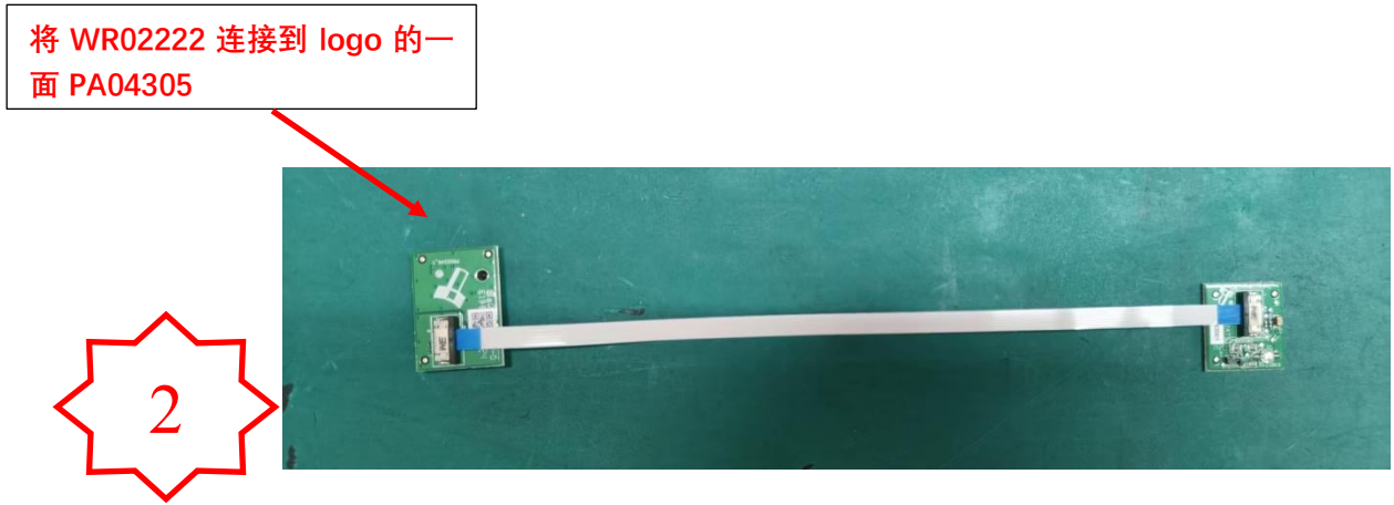
图二，将 WR02222 两端分别插在 PA04305 和 PA04306 PCBA 板的连接器上。
