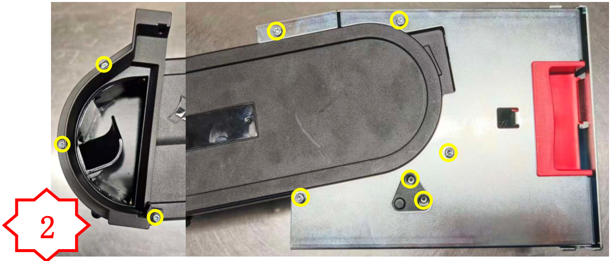
图二，检查三颗 SC119、四颗 SC124 和两颗 SC206 有无漏打。物料表面有无刮花
