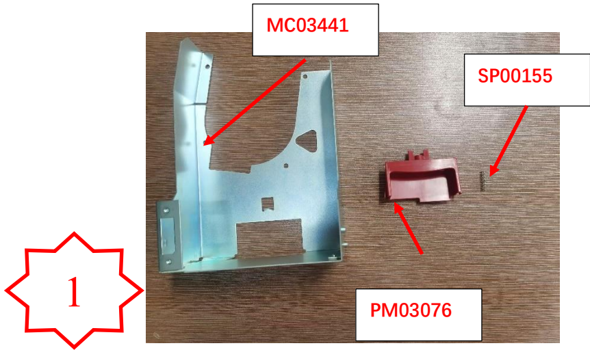
图一，物料识别 MC03441、PM03076、SP00155。
