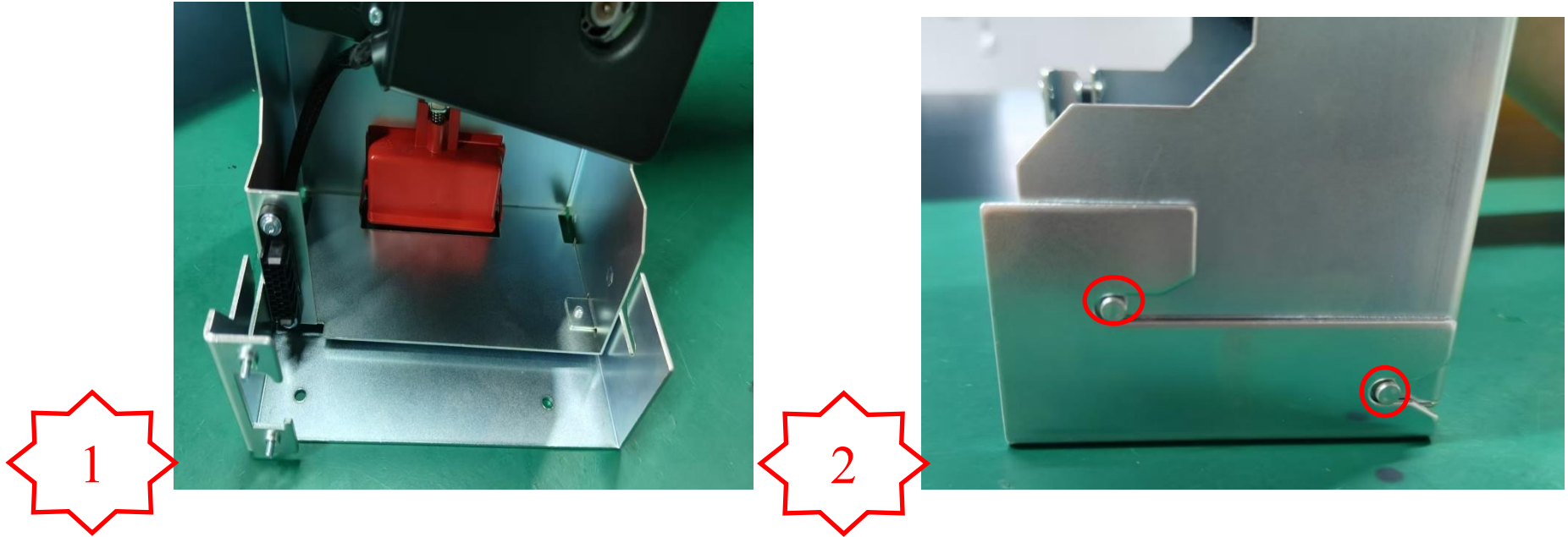
图一, 将 PA03703 装入 PA04401-4 中。
