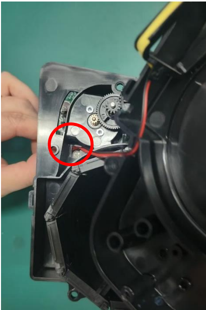
图一，将 PA03668 线从孔中穿过
