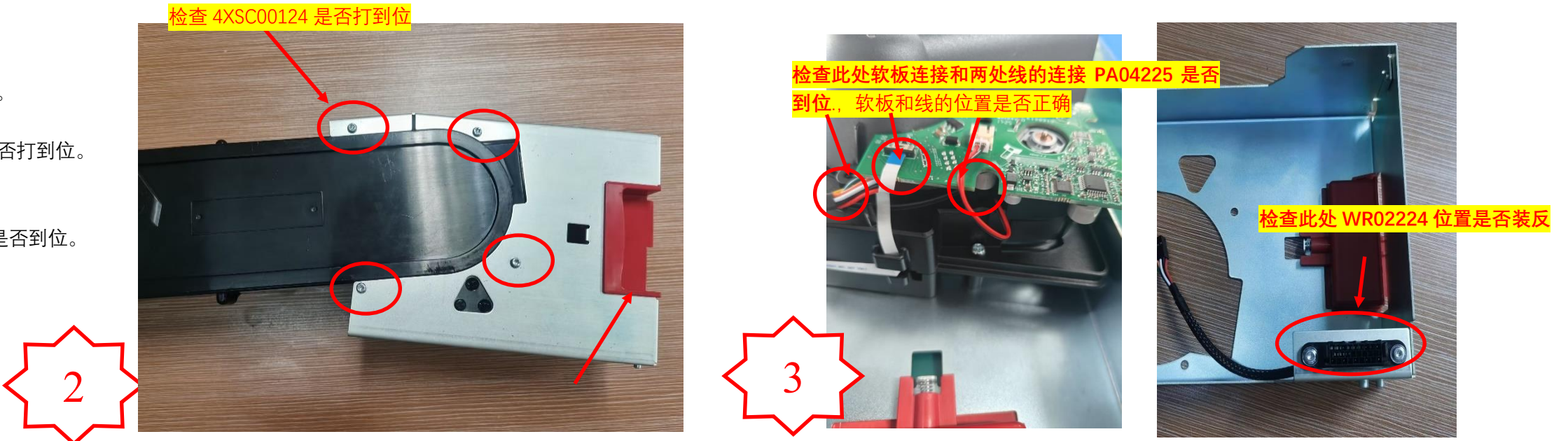
图一，目检 PA04401-3 组件。
