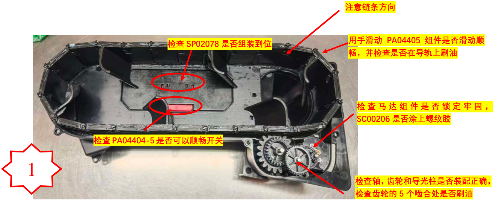
图一, 目检 PA04404-9 组件。
