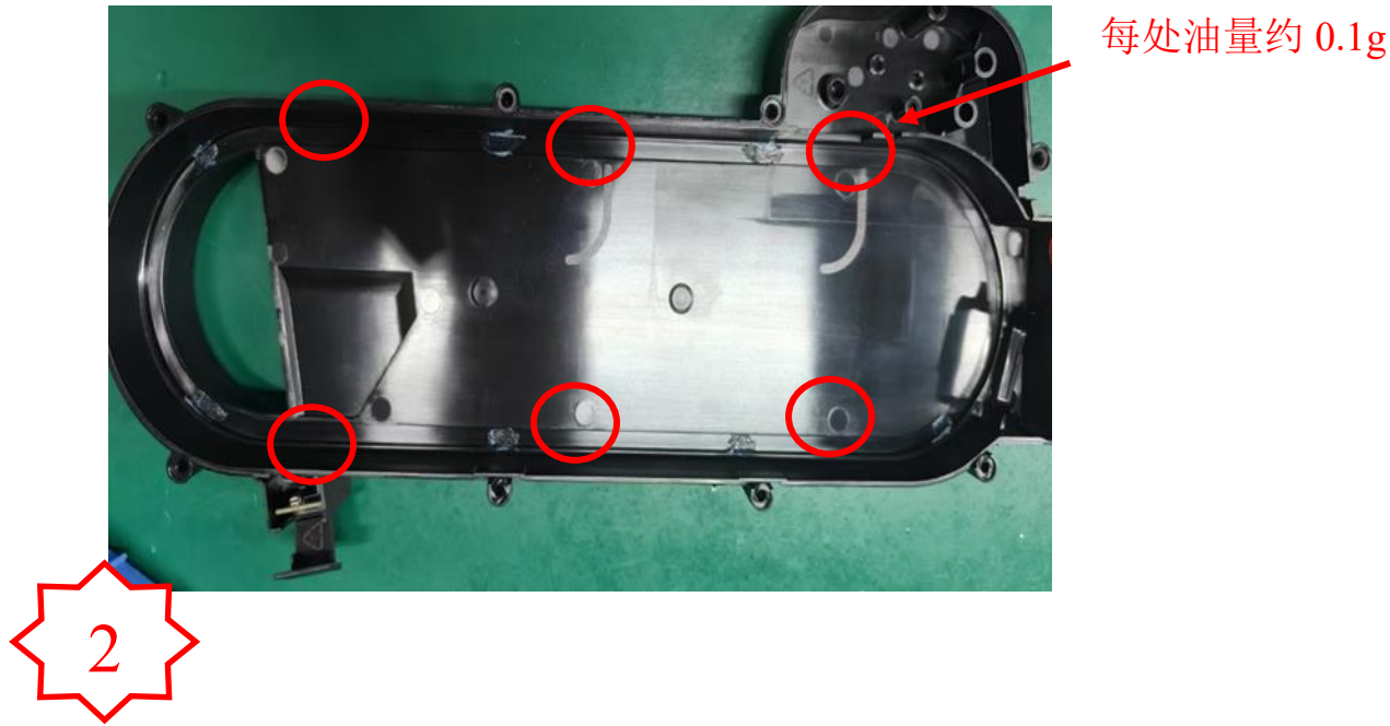
图二, 检查 PM04151 六处点油处是否都点上黄油, 少油或者缺油需手动补充。(PM04152 检查也按照此步骤进行操作)
