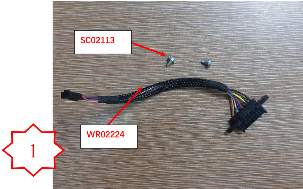
图一, 物料识别 WR02224 和 SC02113。
