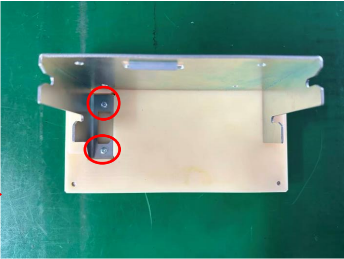
图二，将两颗 SC00116 锁进 MC02466 红圈所示位置，该螺丝为松配
