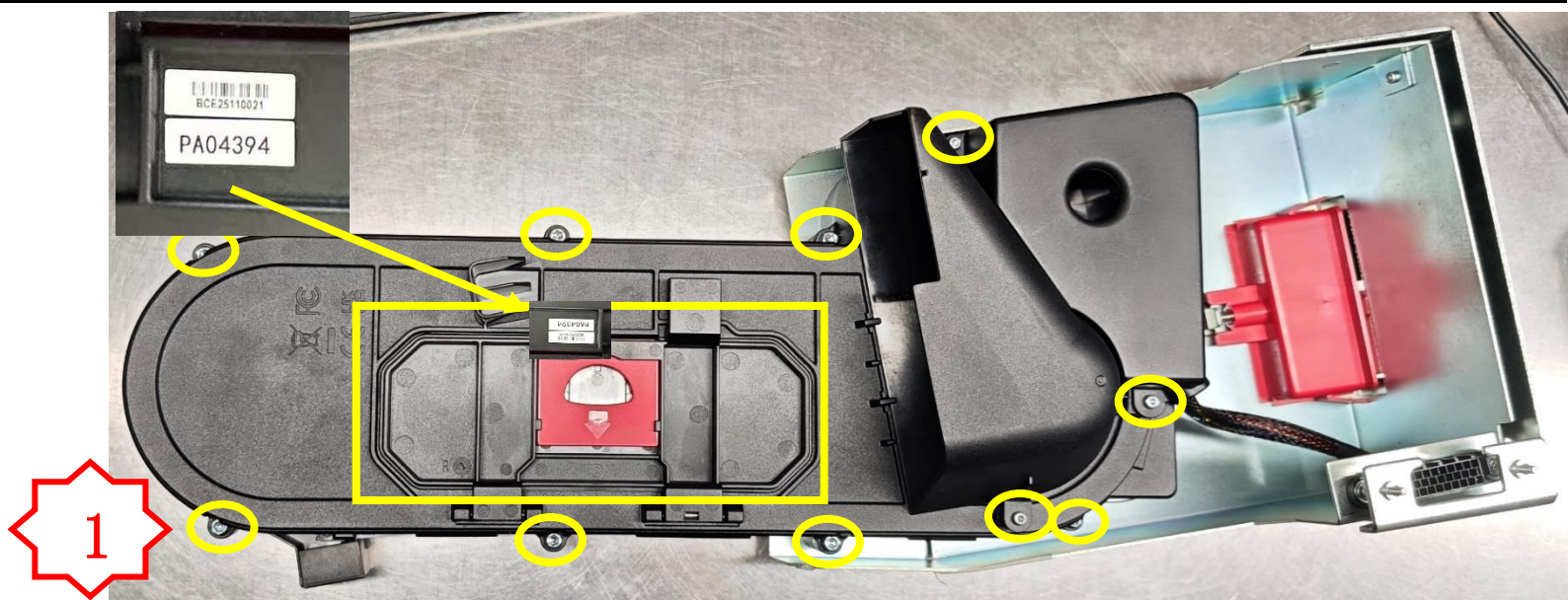
图一，检查七颗 SC124 和三颗 SC119 的螺丝有无漏打，以及窗口打开是否顺畅。注意是否漏贴条码标签和型号标签。
