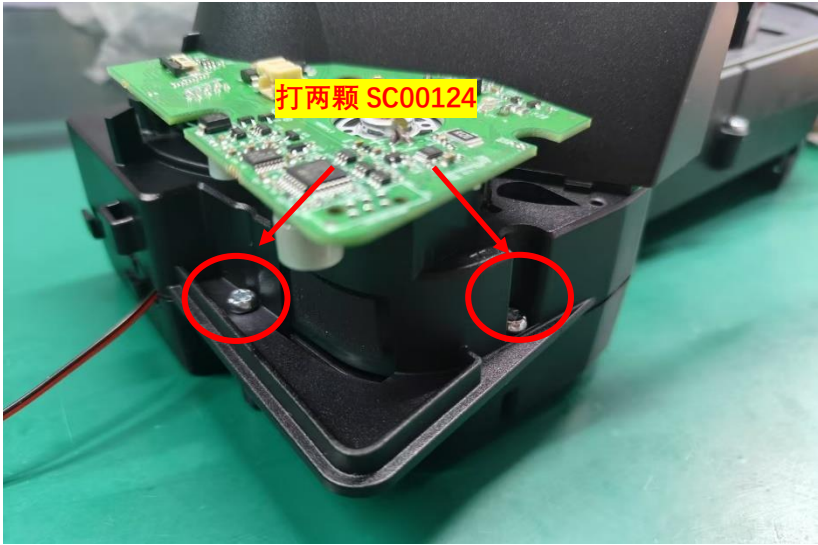
图一, PA04403-3 组件红圈位置打两颗 SC00124。
