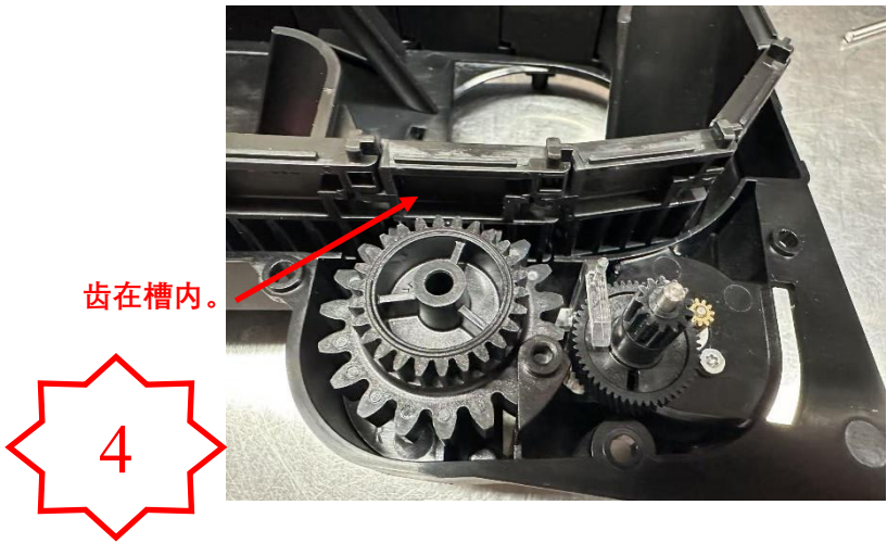
图四, 将 PM03945 装在 PA04404-6 上, 确认 PM03945 的齿与 PA04405-2 组件槽配合
