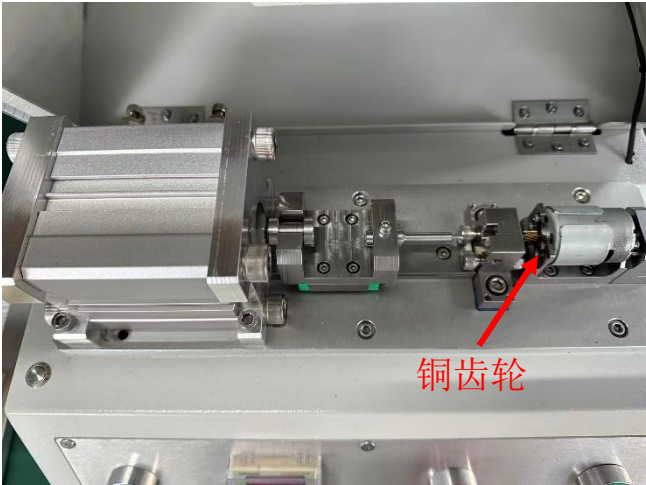
图一, 用马达气动压合治具将 MR02023 与 MC03309 进行压合
