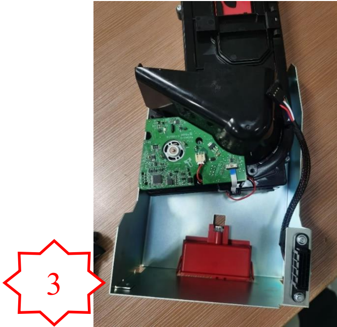
图三, 将装配好的组件翻转 180°。
